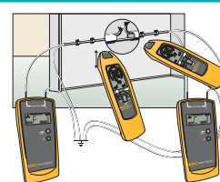
Localizare precisă a întreruperilor cu un emițător suplimentar
